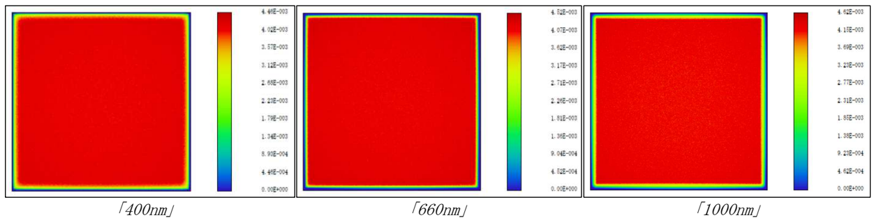
〈同一作動距離でのフォーカス状態（3波長で同一視野範囲を計算）〉
